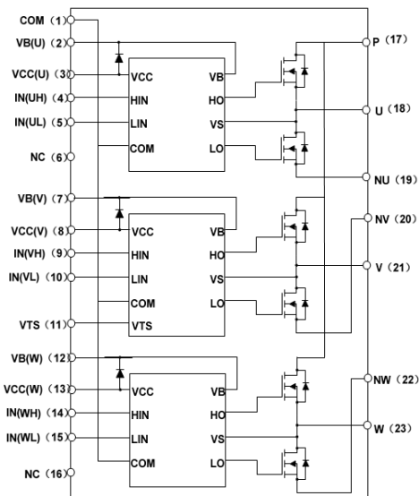
图 1：模块内部电路示意图
