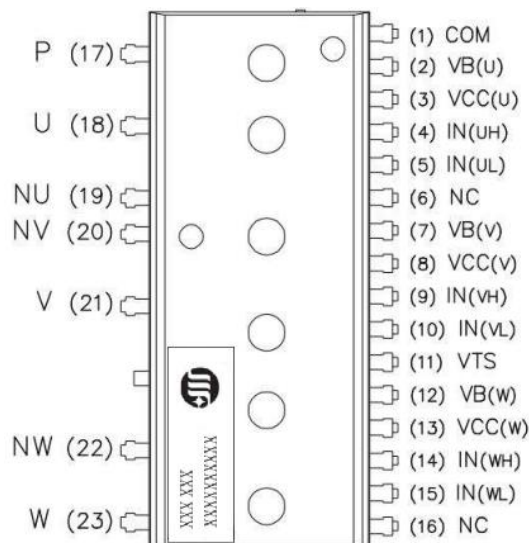
图 2：模块引脚分布示意图
