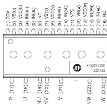
PIN1-PIN23
