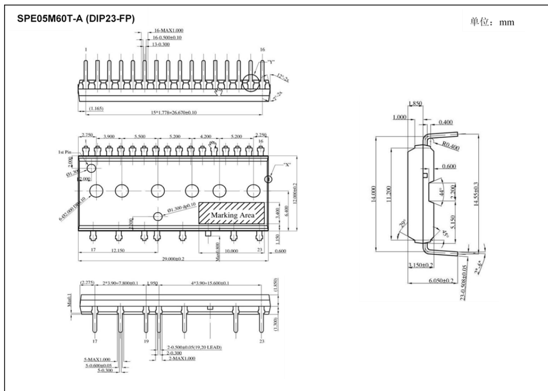
图 11: SPE05M60T-A 封装外形图
